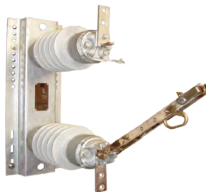
Cuchilla Monopolar Loadbuster Disconnects estilo Branch Feeder (para derivaciones)
